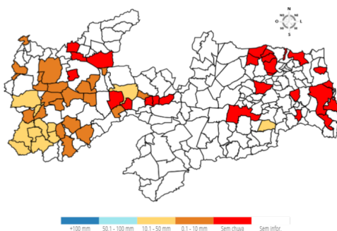
PRECIPITAÇÃO MÁXIMA DOS MUNICÍPIOS/POSTOS NO DIA 11/03/2025
