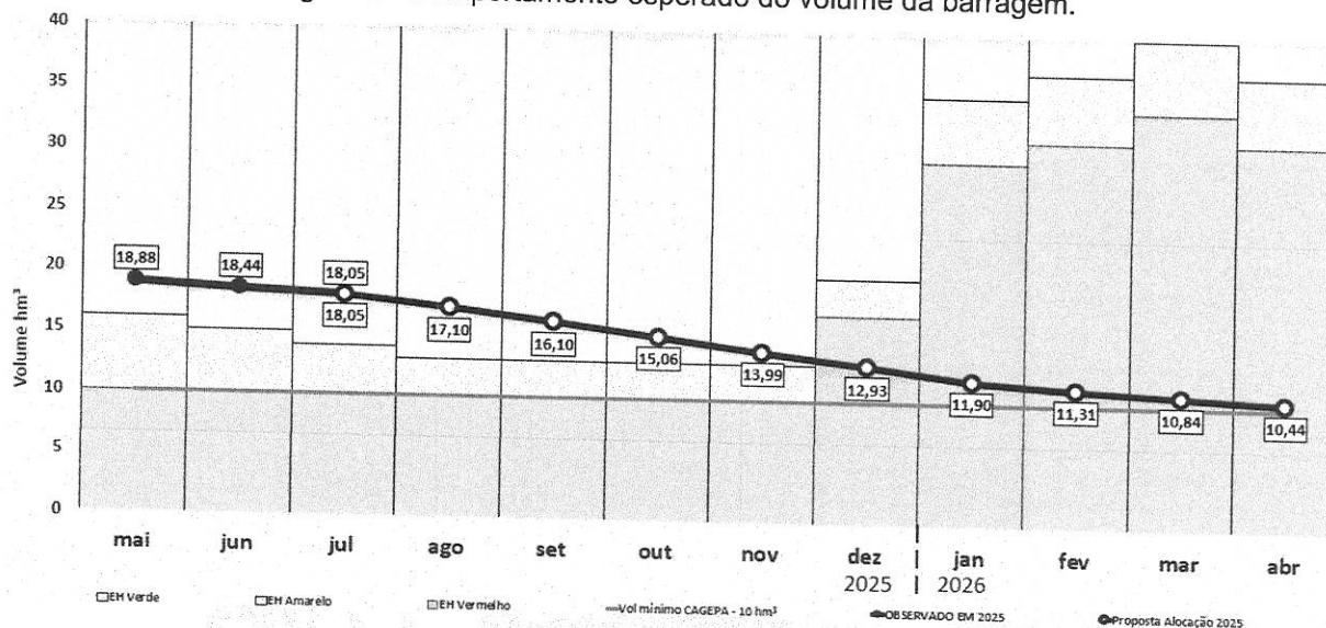
Figura 2 - Comportamento esperado do volume da barragem.
