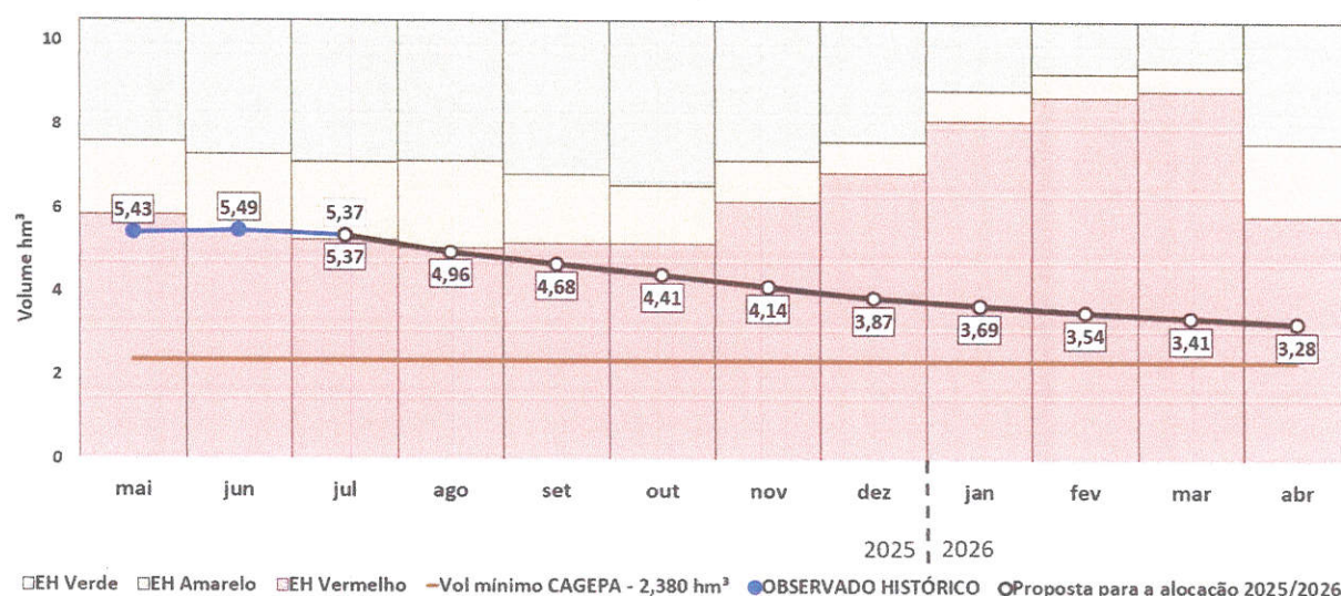
Figura 2 - Comportamento esperado do volume da barragem.
