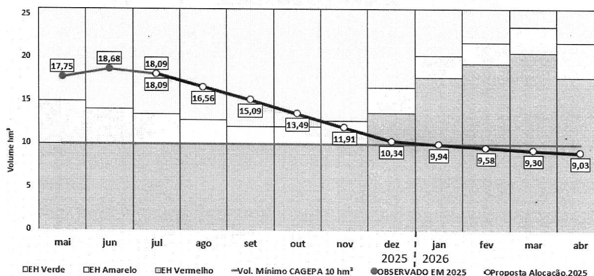
Figura 2 - Comportamento esperado do volume da barragem.
