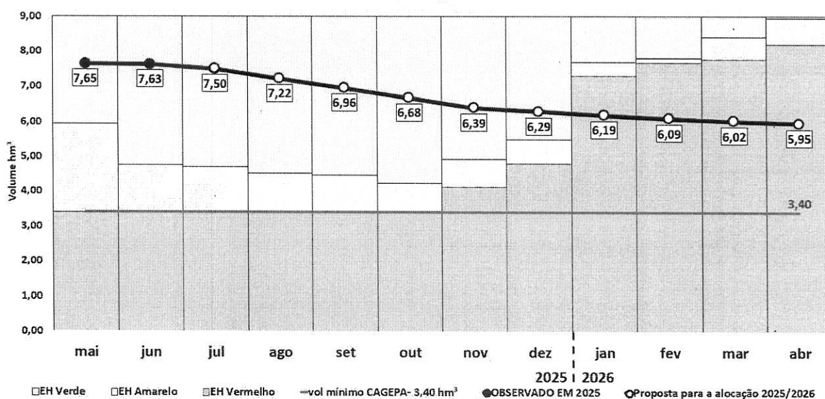
Figura 2 - Comportamento esperado do volume da barragem.
