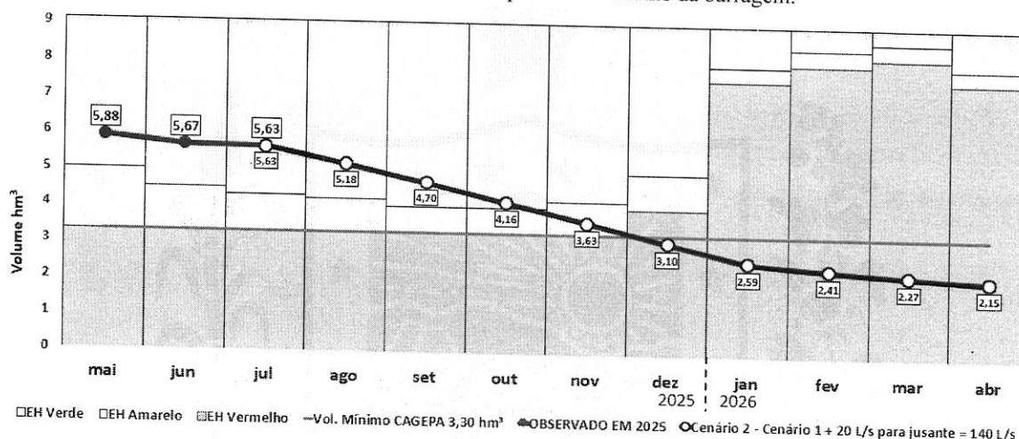
Figura 2 - Comportamento esperado do volume da barragem.
