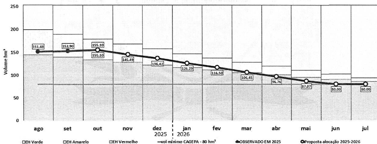
Figura 1 - Comportamento esperado do volume da barragem.
