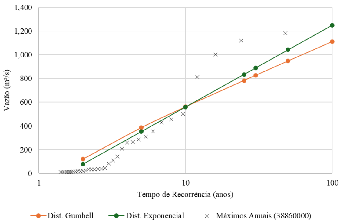
Figura 4.31 - Ajuste das distribuições de Gumbell e Exponencial para a estação 38860000
