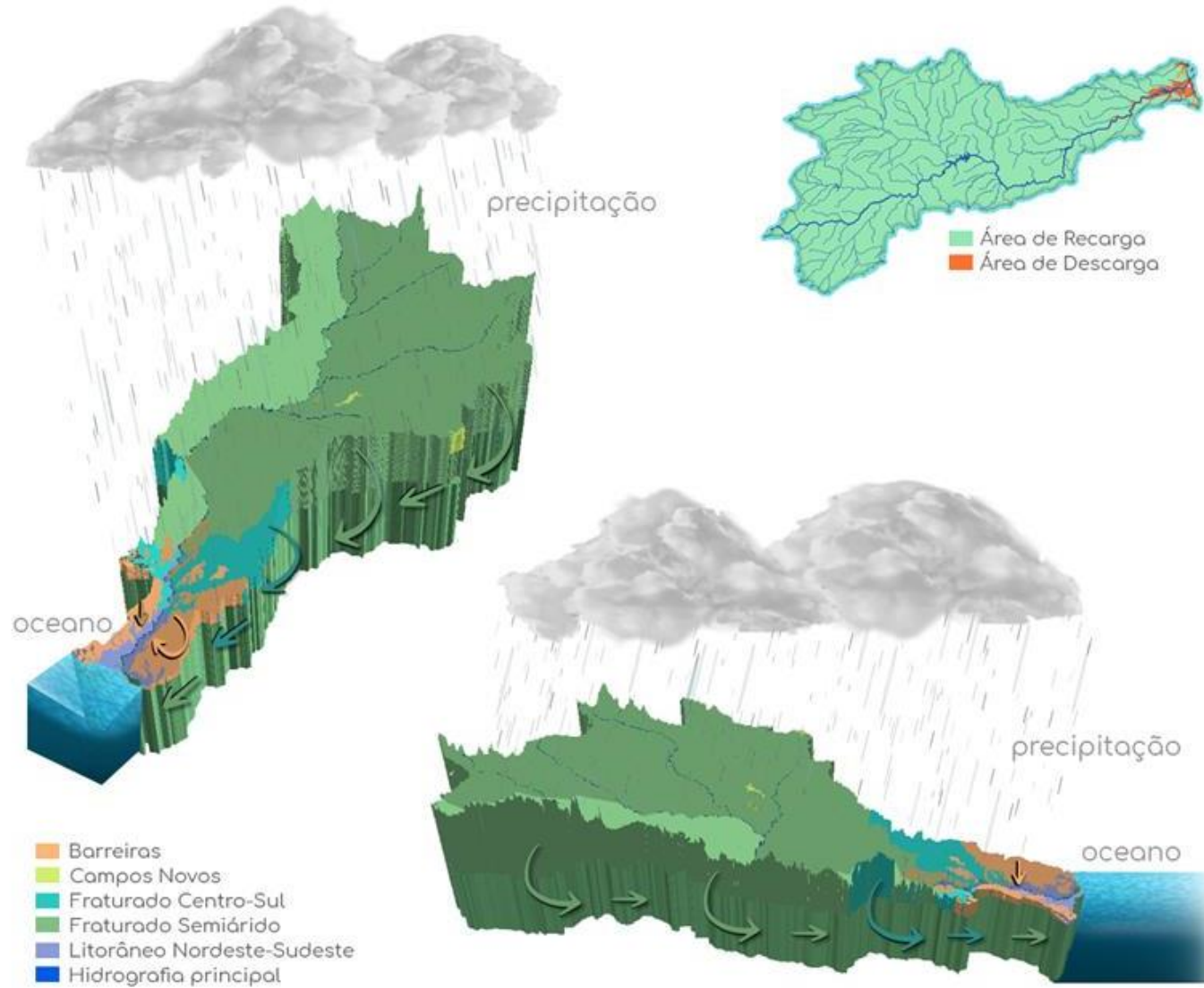
Figura 4.102 - Modelo de Circulação das Águas Subterrâneas na bacia hidrográfica
