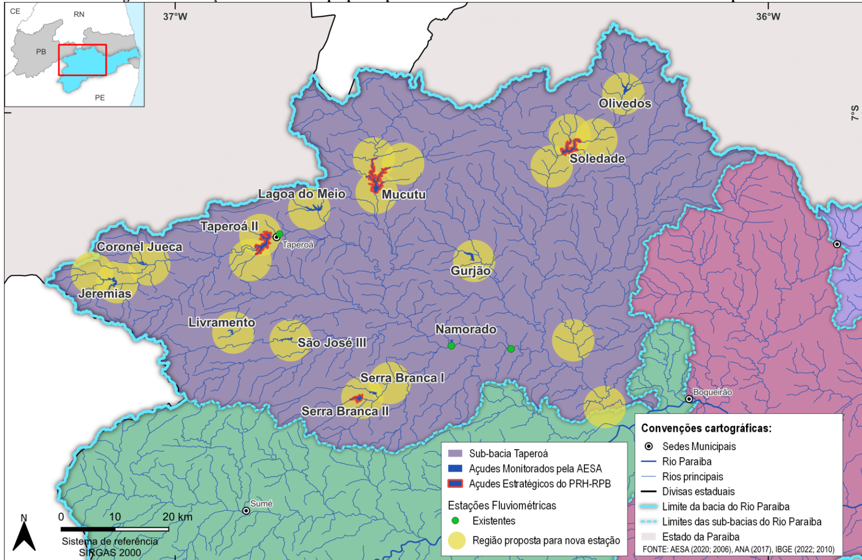
Figura 4.43 - Estações Fluviométricas propostas para melhoria da rede de monitoramento da sub-bacia do Taperoá
