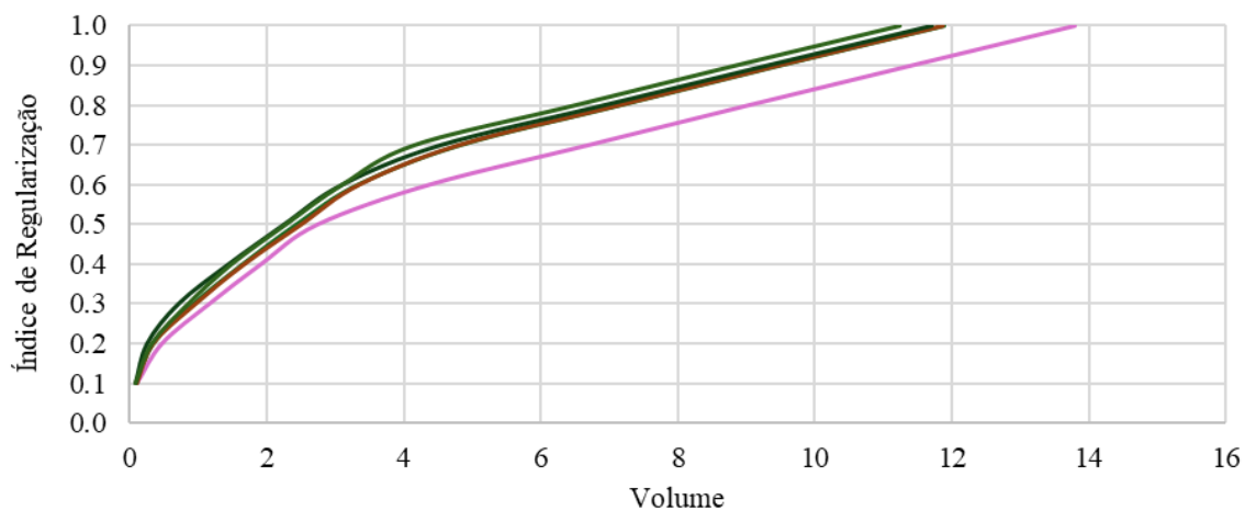
Figura 4.64 - Curvas de Regularização Adimensionais
