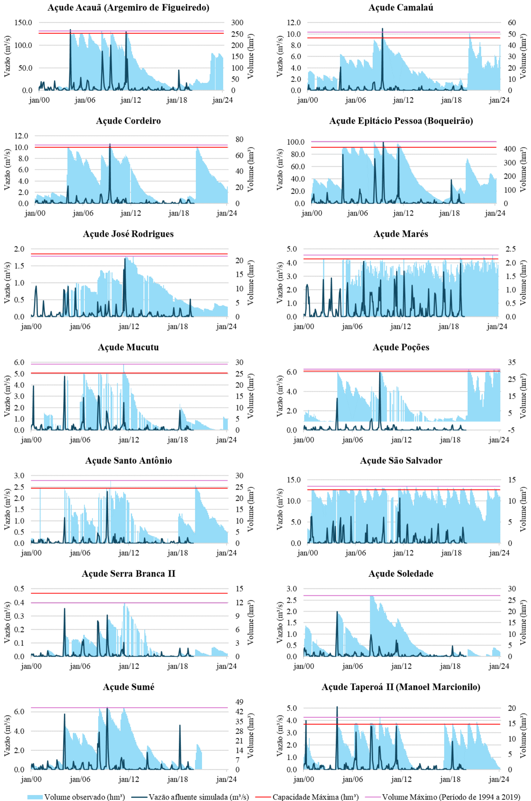
Figura 4.61 - Volumes observados e vazões afluentes simuladas
