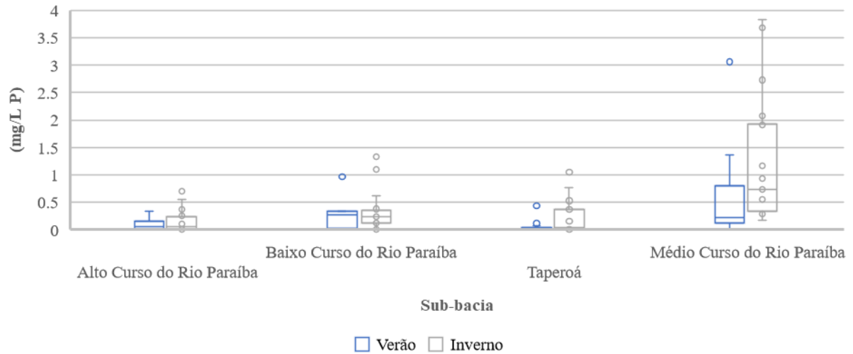
Figura 4.119 - Concentrações médias de ortofosfato por estação do Ano
