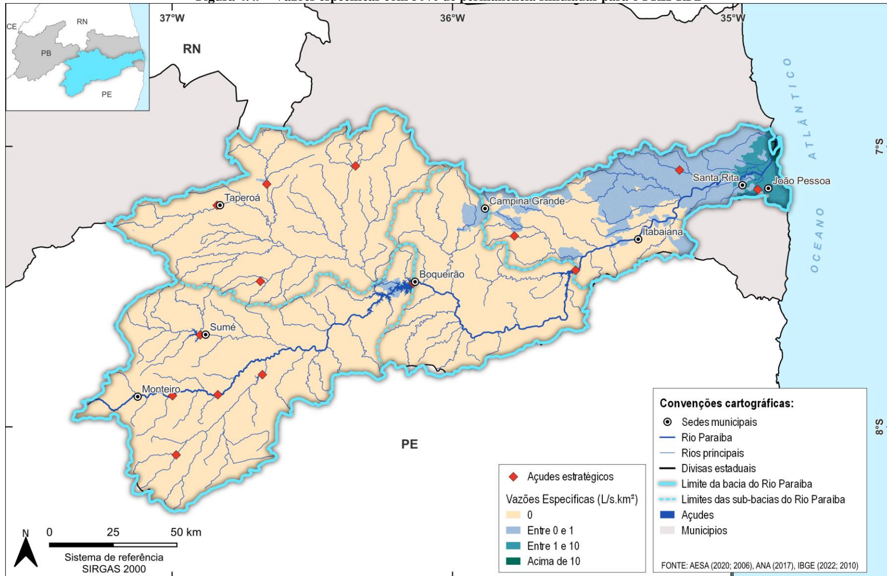
Figura 4.49 - Vazões específicas com 50% de permanência simuladas para o PRH-RPB
