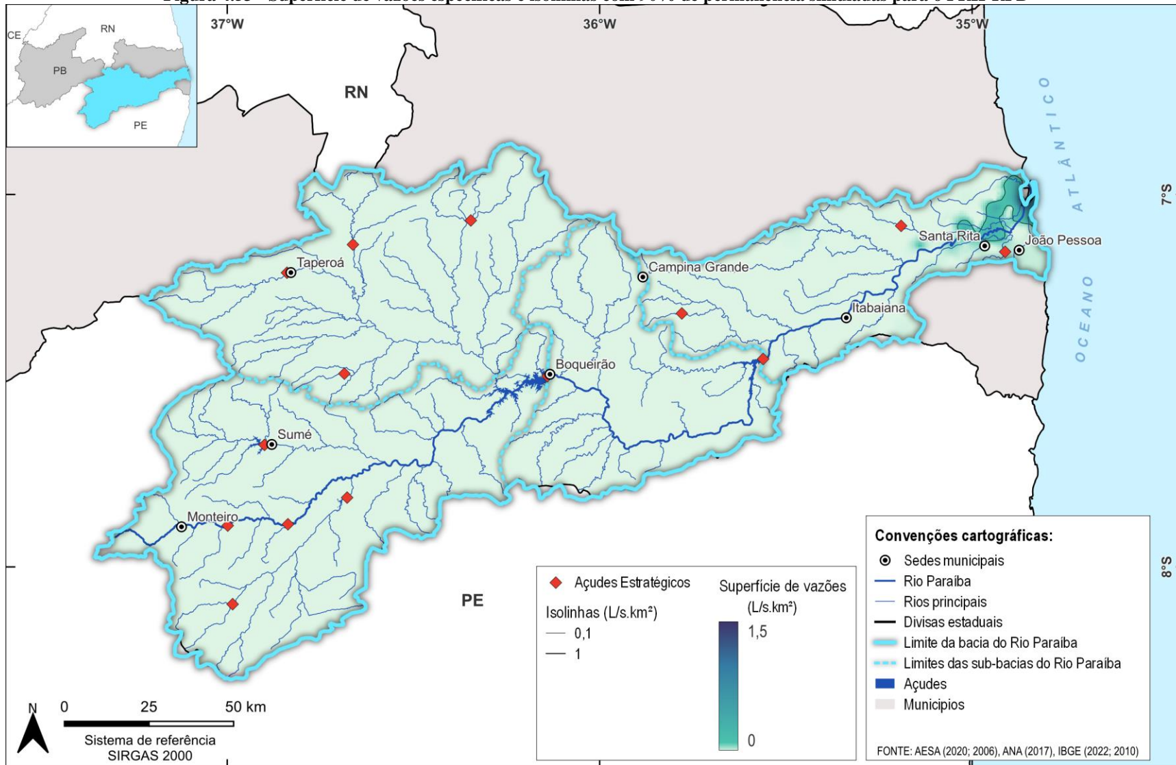
Figura 4.53 - Superfície de vazões específicas e isolinhas com 90% de permanência simuladas para o PRH-RPB
