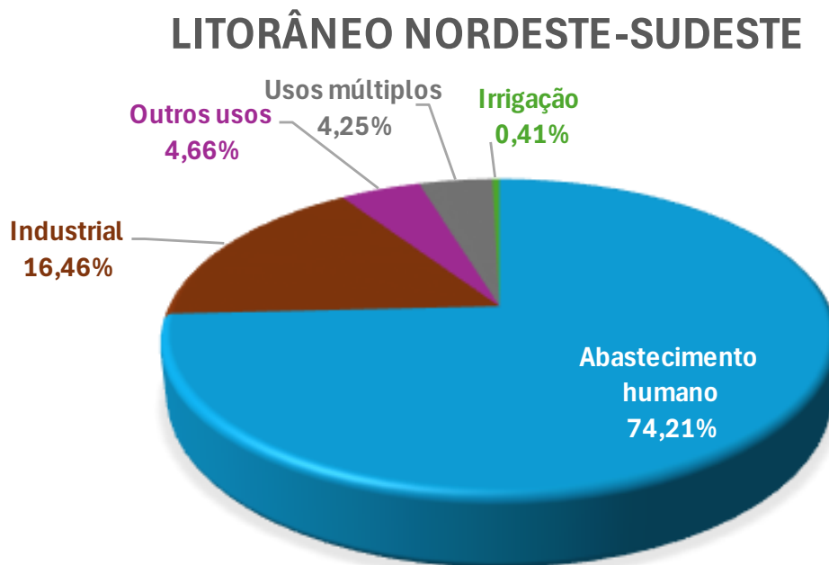
Figura 4.95 - Percentual por tipo de uso, individualizados por Sistema Aquífero - Litorâneo Nordeste-Sudeste
