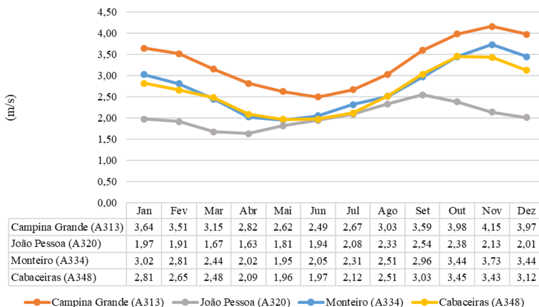
Figura 4.8 - Velocidade média do vento registrado nas estações automáticas
