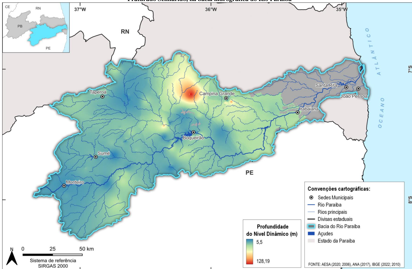
Figura 4.78 - Superfície Potenciométrica representando as Cotas (em relação ao nível médio do mar) dos Níveis Dinâmicos dos poços tubulares do sistema aquífero Fraturado Semiárido, na bacia hidrográfica do Rio Paraíba
