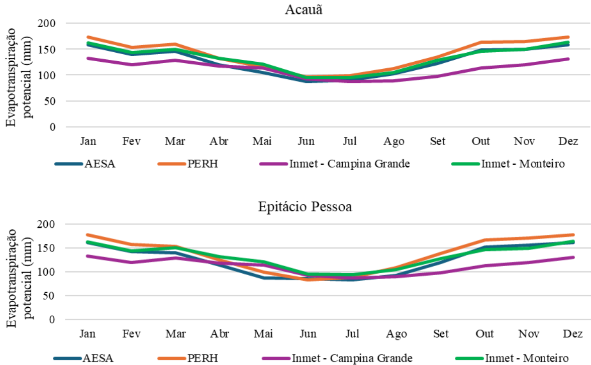
Figura 4.15 - Evapotranspiração potencial estimada para os açudes de Acauã e Epitácio Pessoa
