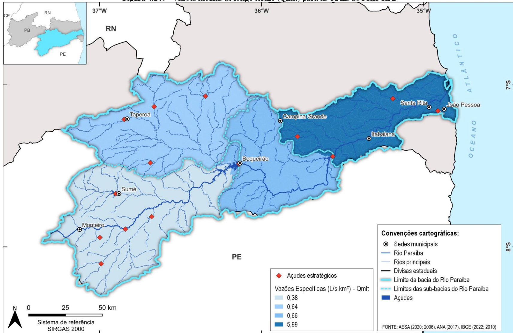
Figura 4.140 - Vazões médias de longo termo (Q mt ) para as UPHs do PRH-RPB
