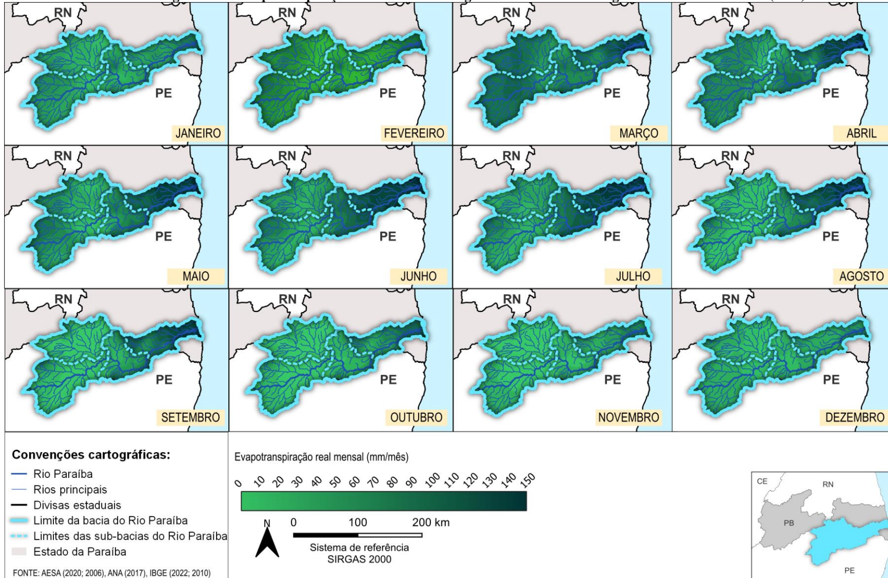
Figura 4.17 - Evapotranspiração real da bacia hidrográfica do Rio Paraíba segundo Francisco & Santos (2017)
