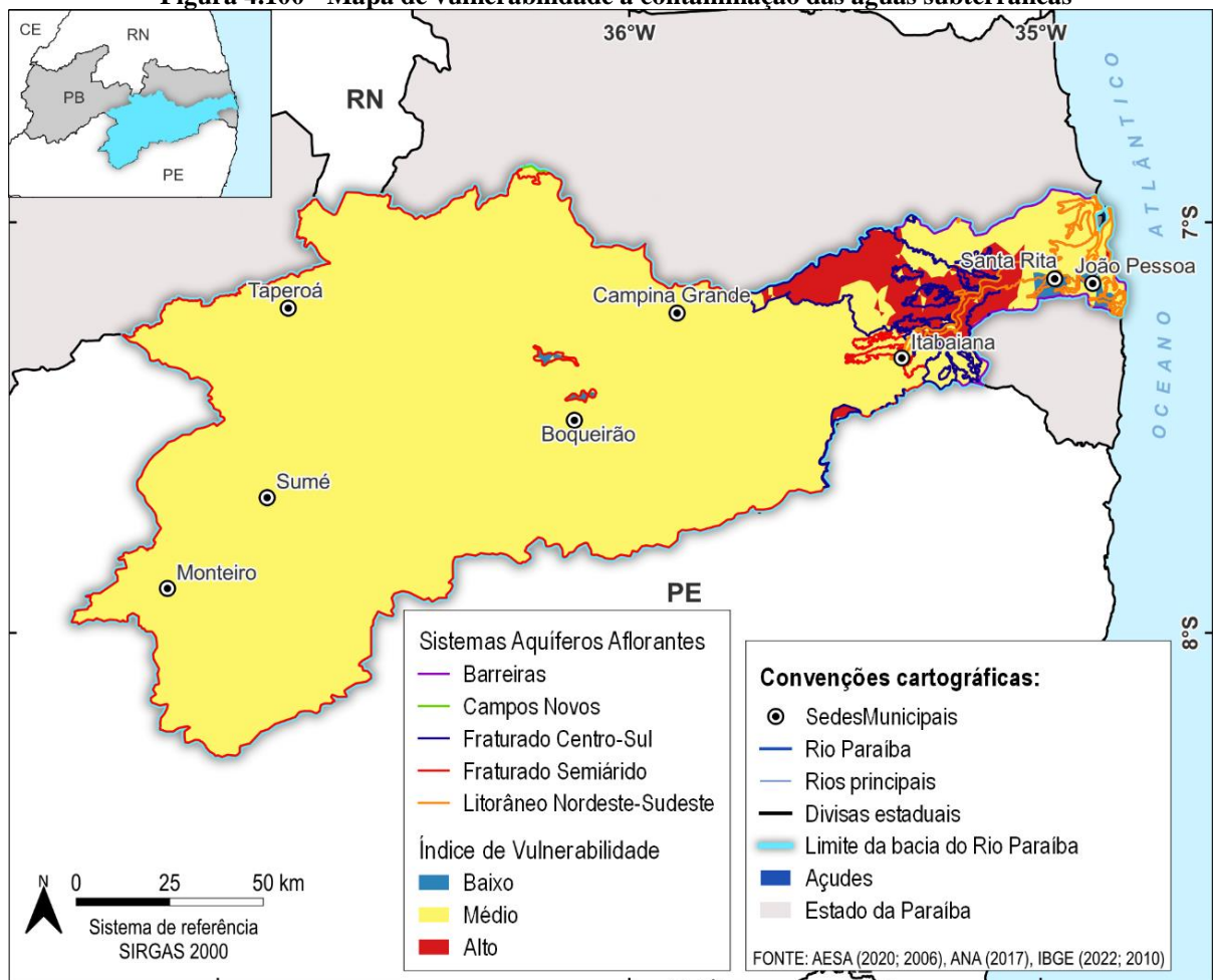
Figura 4.100 - Mapa de vulnerabilidade à contaminação das águas subterrâneas
