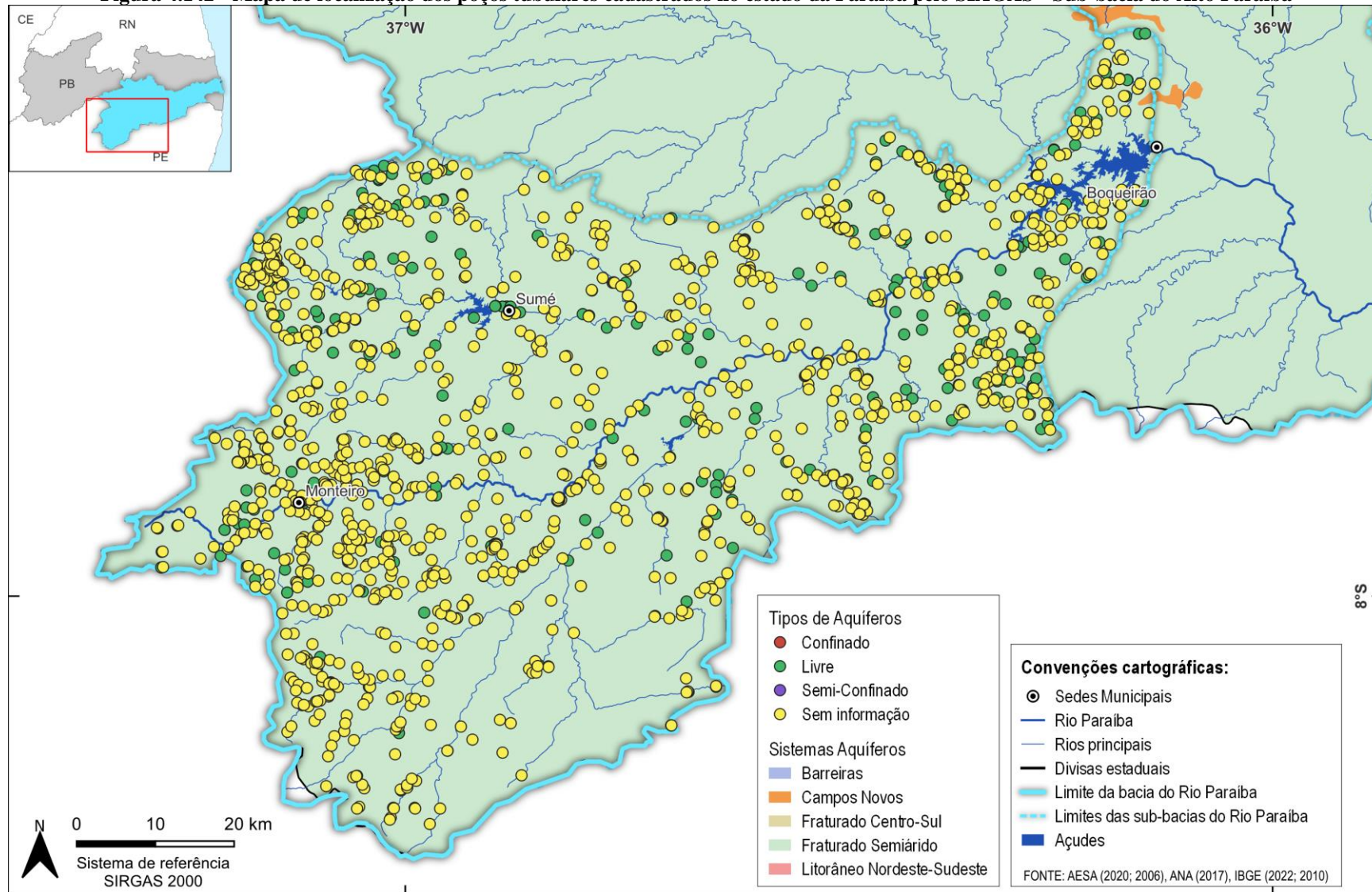
Figura 4.142 - Mapa de localização dos poços tubulares cadastrados no estado da Paraíba pelo SIAGAS - Sub-bacia do Alto Paraíba
