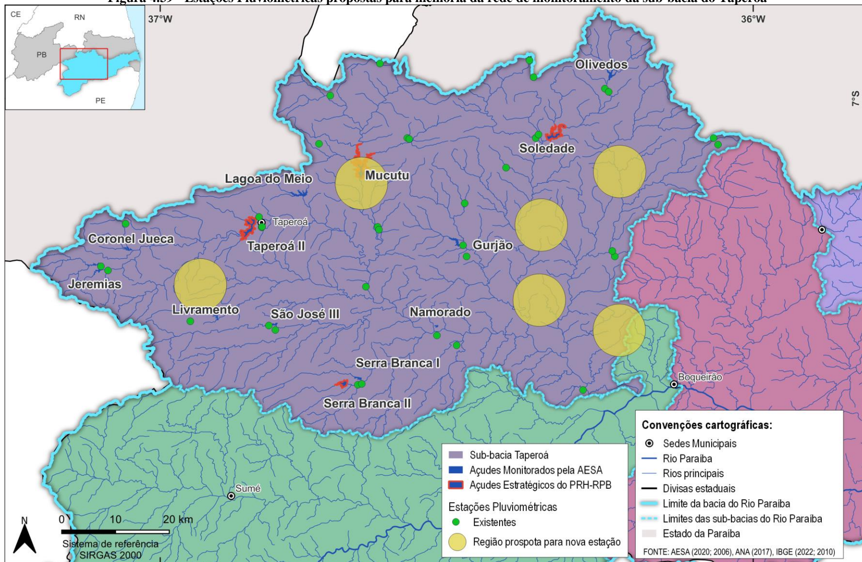
Figura 4.39 - Estações Pluviométricas propostas para melhoria da rede de monitoramento da sub-bacia do Taperoá
