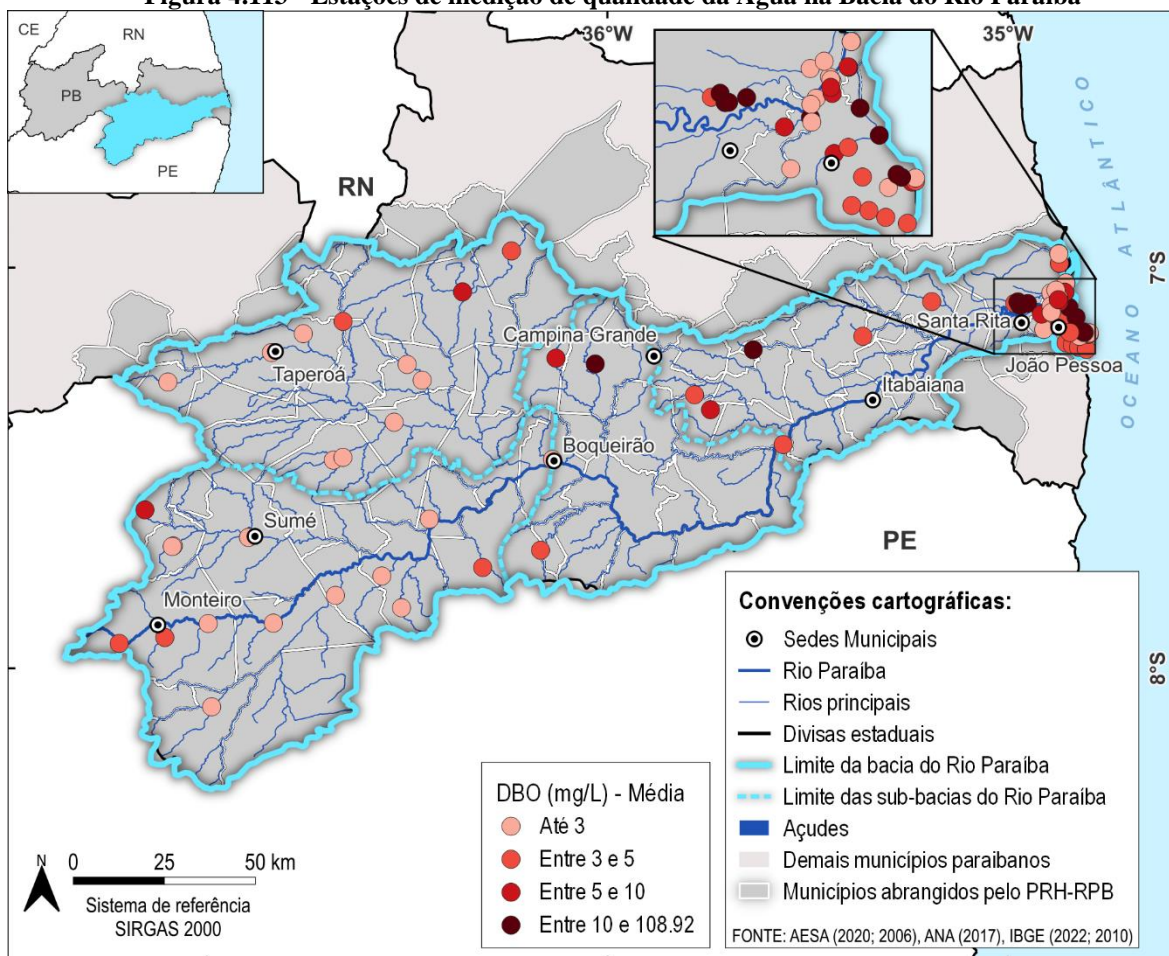
Figura 4.113 - Estações de medição de qualidade da Água na Bacia do Rio Paraíba
