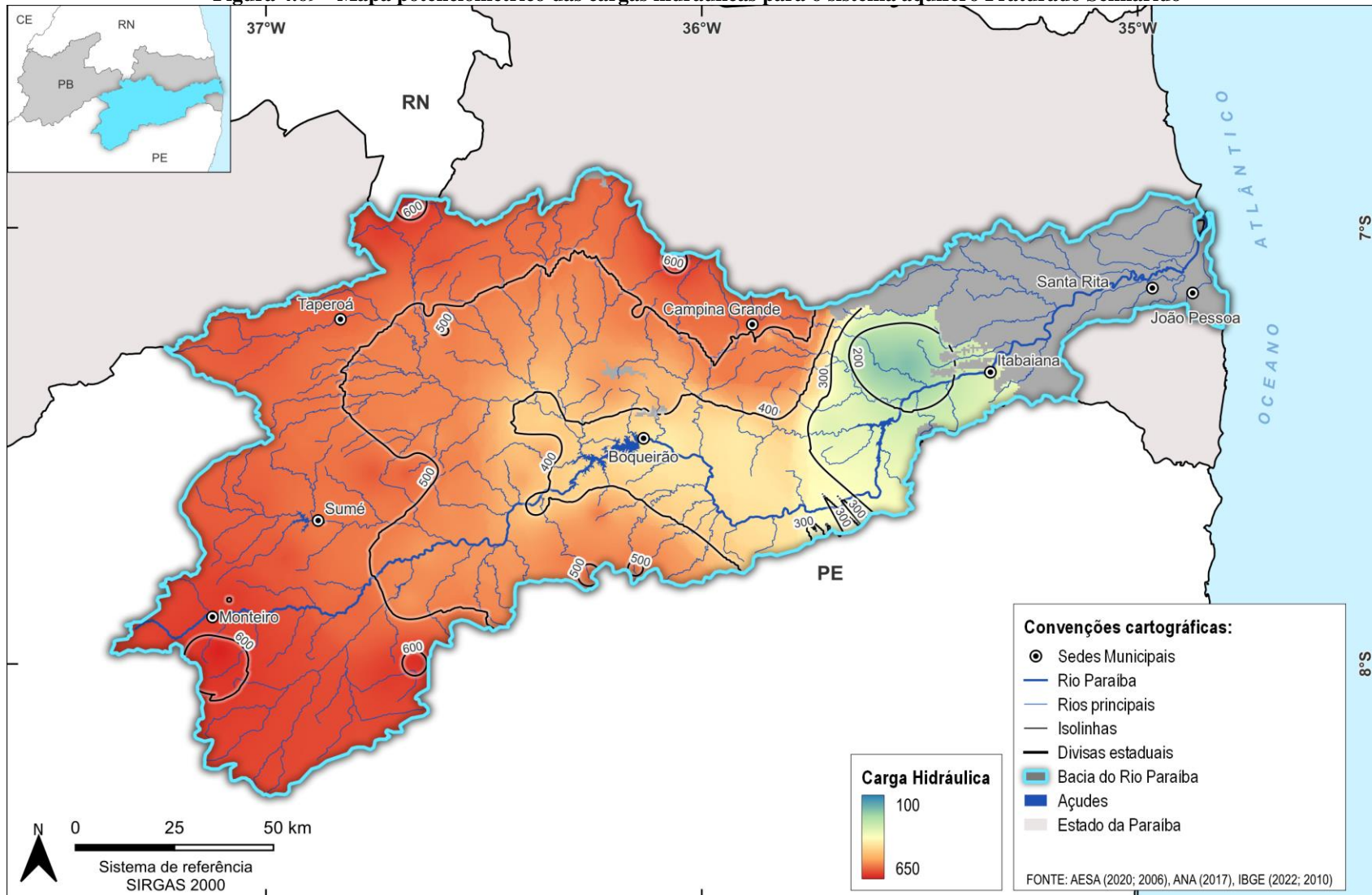
Figura 4.69 - Mapa potenciométrico das cargas hidráulicas para o sistema aquífero Fraturado Semiárido
