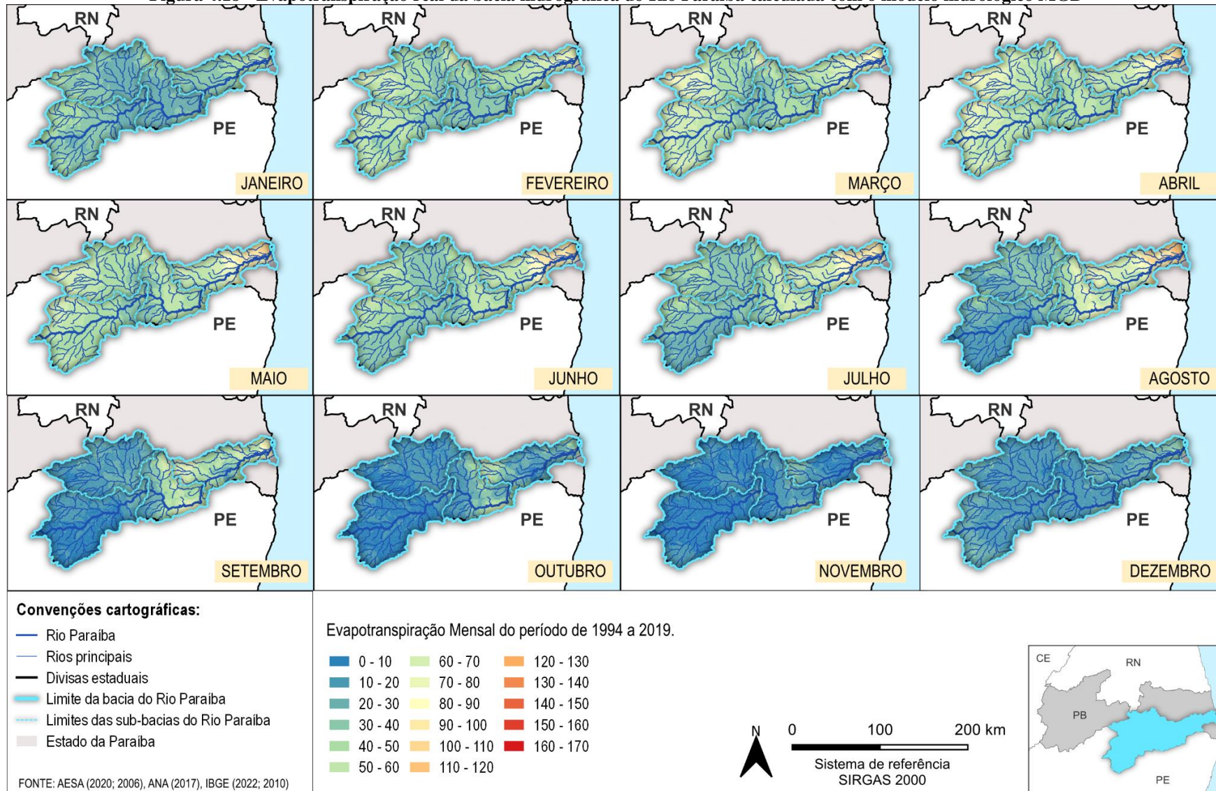
Figura 4.18 - Evapotranspiração real da bacia hidrográfica do Rio Paraíba calculada com o modelo hidrológico MGB
