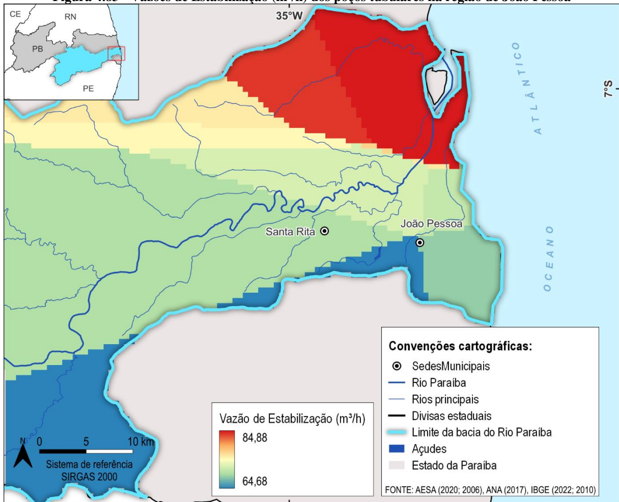
Figura 4.83 - Vazões de Estabilização ( m^3/h ) dos poços tubulares na região de João Pessoa
