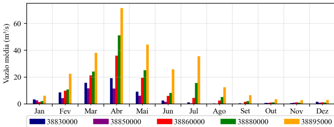
Figura 4.26 - Variação sazonal das vazões médias mensais
