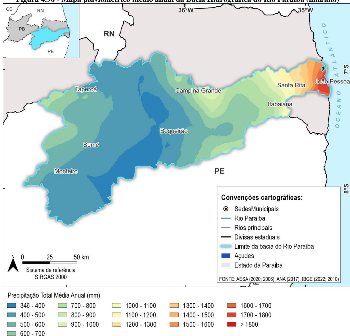
Figura 4.96 - Mapa pluviométrico médio anual da Bacia Hidrográfica do Rio Paraíba (mm/ano)
