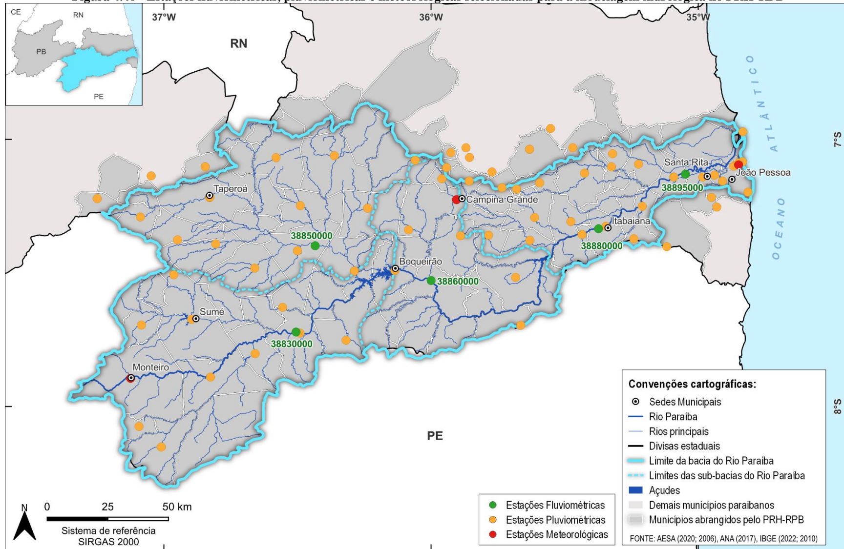
Figura 4.46 - Estações fluviométricas, pluviométricas e meteorológicas selecionadas para a modelagem hidrológica no PRH-RPB
