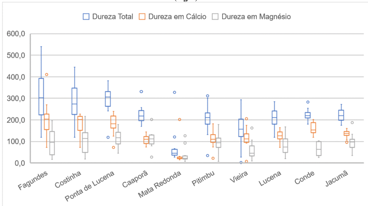
Figura 4.132 - Distribuição nos valores de concentração de dureza nos poços monitorados pela CAGEPA (mg/L)
