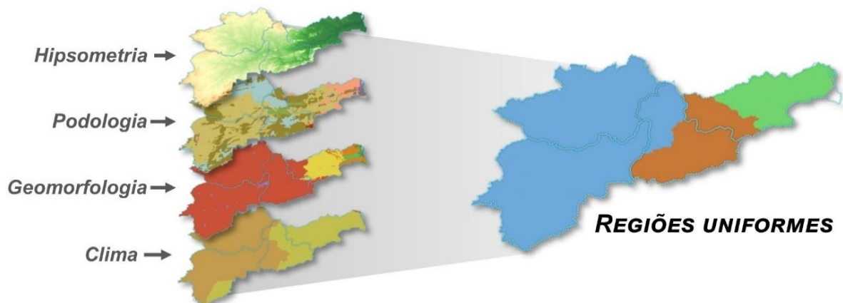
Figura 4.45 - Regiões com características uniformes da Bacia do Rio Paraíba
