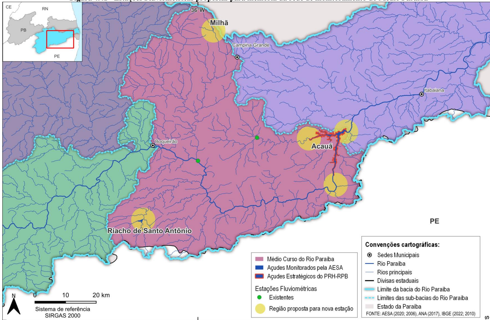
Figura 4.41 - Estações Fluviométricas propostas para melhoria da rede de monitoramento do Médio Paraíba
