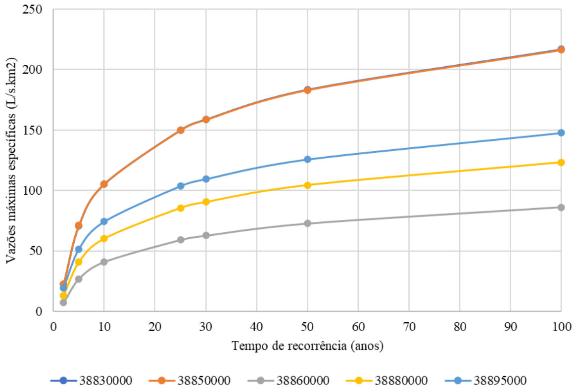
Figura 4.34 - Vazões máximas específicas (L/s.km 2 ) - média dos ajustes
