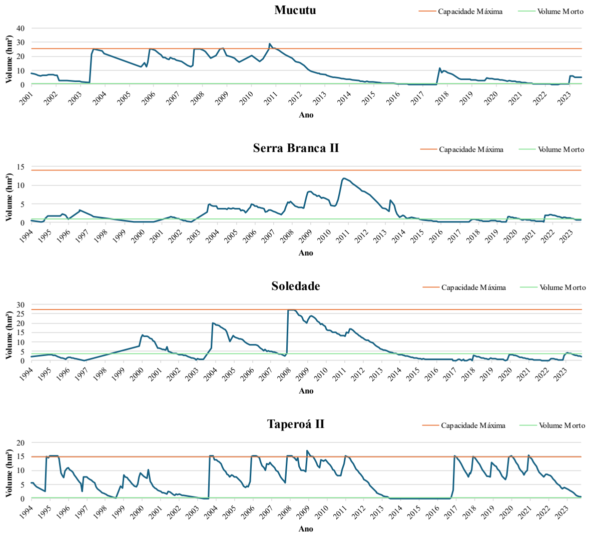
Figura 4.60 - Série histórica de volume dos reservatórios estratégicos da sub-bacia Taperoá em hm 3
