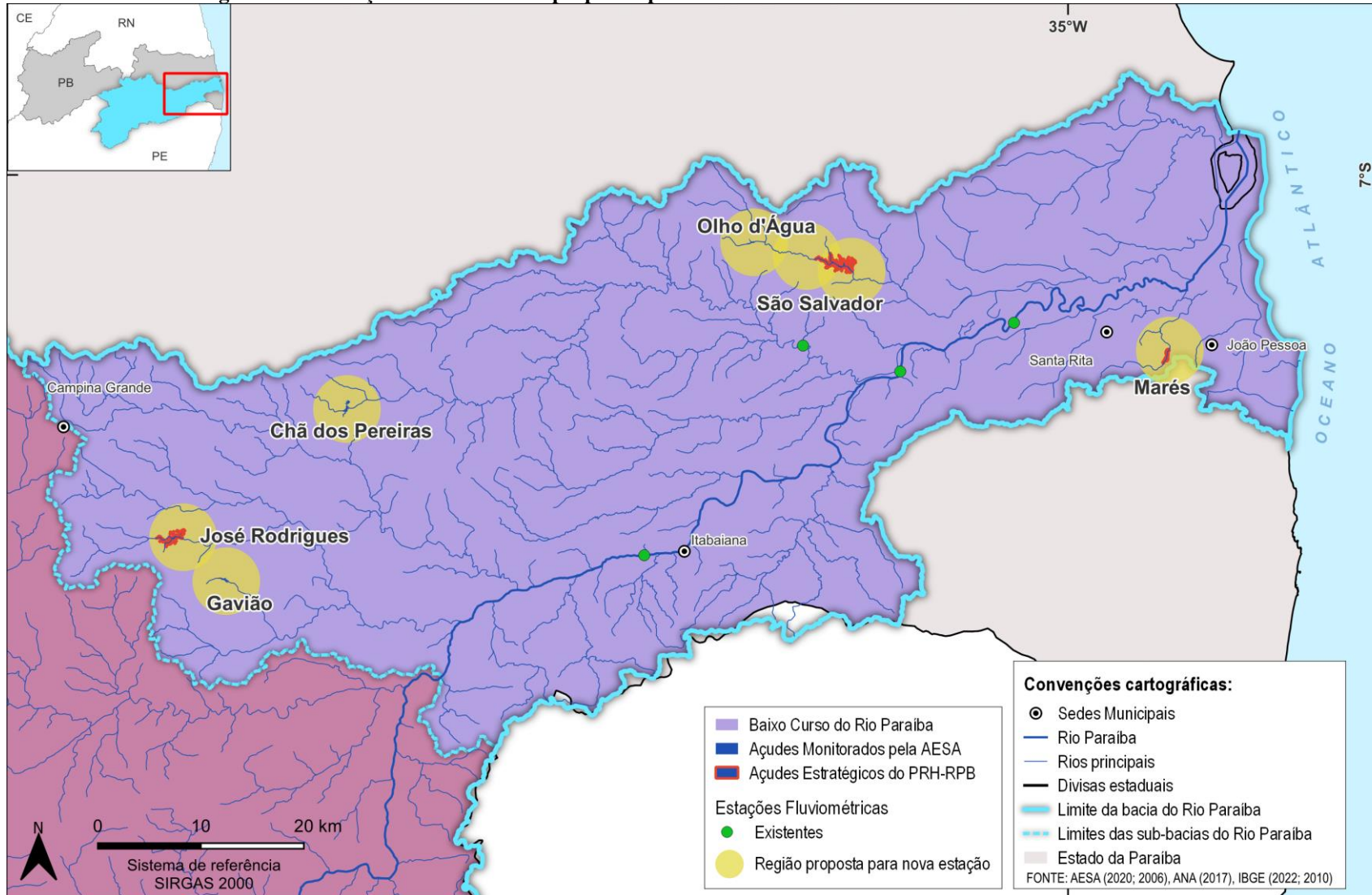
Figura 4.42 - Estações Fluviométricas propostas para melhoria da rede de monitoramento do Baixo Paraíba
