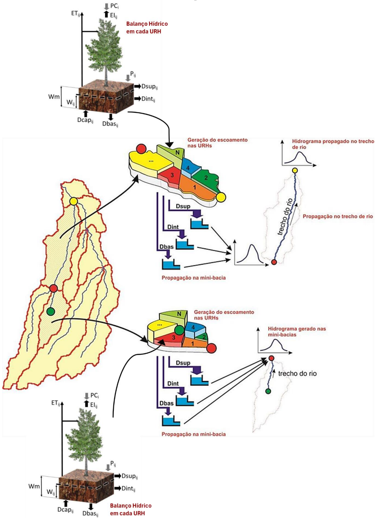
Figura 4.44 - Esquema do MGB
