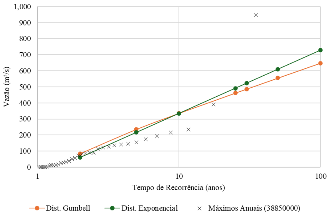
Figura 4.30 - Ajuste das distribuições de Gumbell e Exponencial para a estação 38850000
