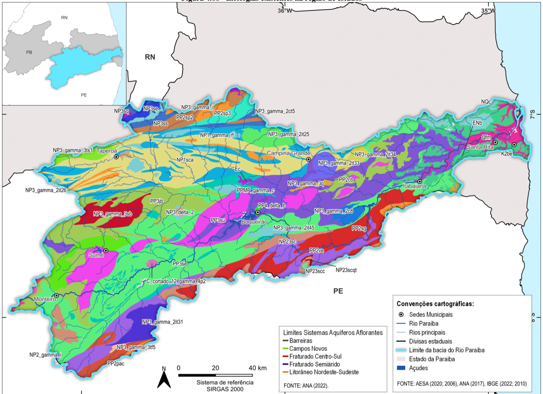
Figura 4.66 - Litologias existentes na região de estudos
