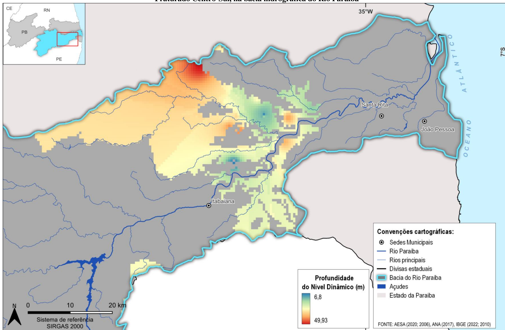
Figura 4.79 - Superfície Potenciométrica representando as Cotas (em relação ao nível médio do mar) dos Níveis Dinâmicos dos poços tubulares do sistema aquífero Fraturado Centro-Sul, na bacia hidrográfica do Rio Paraíba
