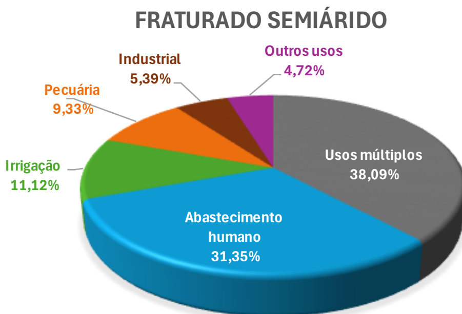
Figura 4.94 - Percentual por tipo de uso, individualizados por Sistema Aquífero - Fraturado Semiárido
