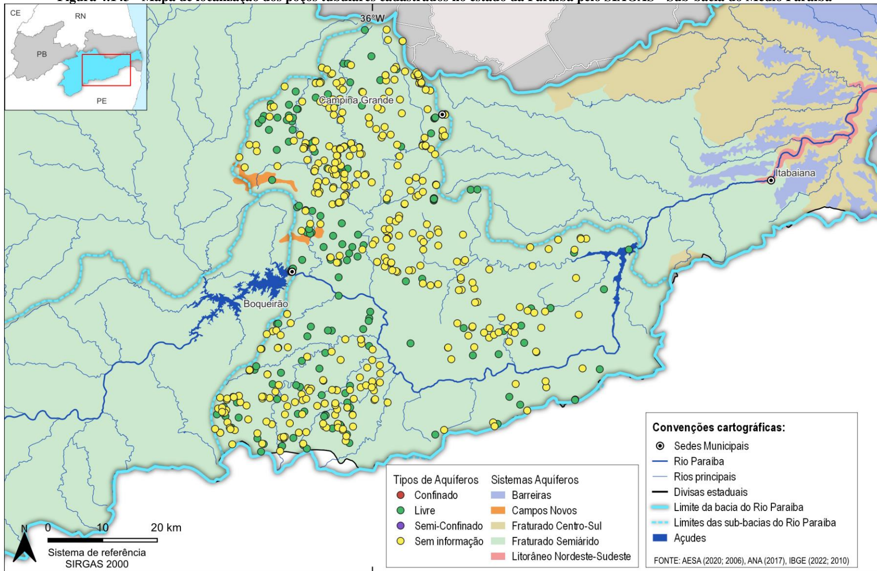
Figura 4.143 - Mapa de localização dos poços tubulares cadastrados no estado da Paraíba pelo SIAGAS - Sub-bacia do Médio Paraíba
