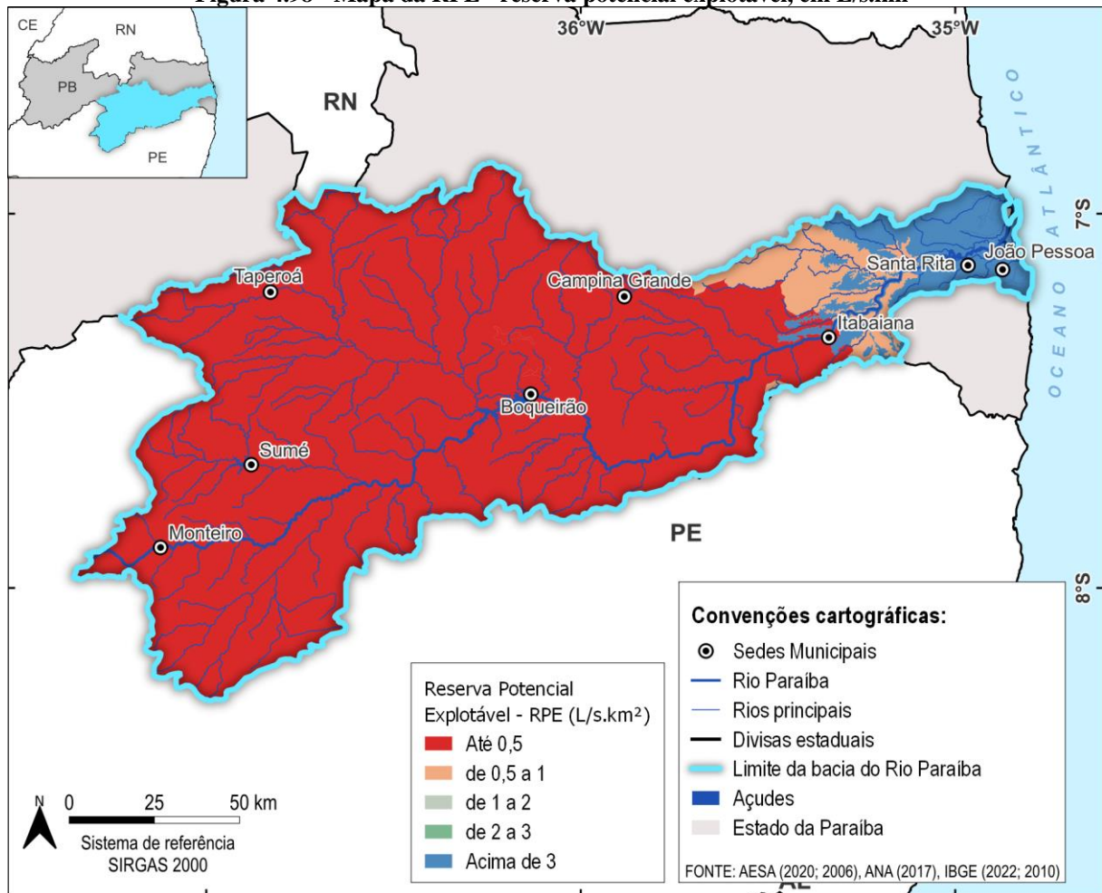
Figura 4.98 - Mapa da RPE - reserva potencial explotável, em L/s.km 2
