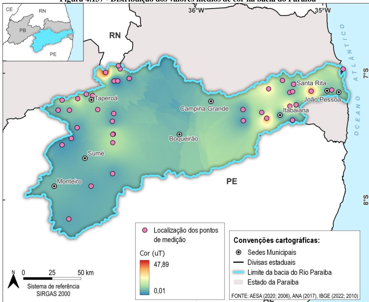
Figura 4.137 - Distribuição dos valores médios de cor na bacia do Paraíba
