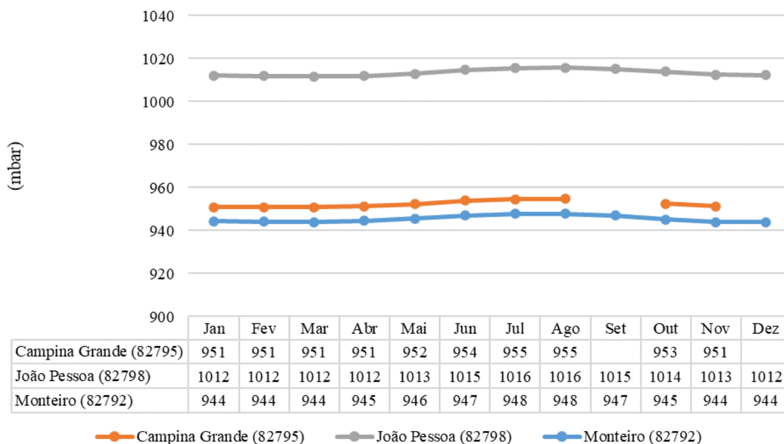
Figura 4.11 - Pressão atmosférica média mensal registrada nas estações convencionais
