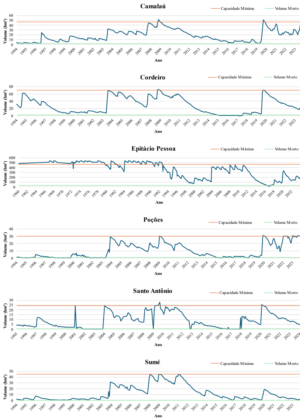
Figura 4.57 - Série histórica de volume dos reservatórios estratégicos do Alto Paraíba
