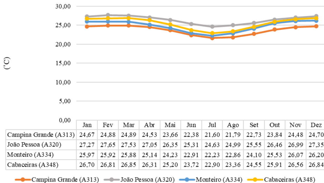
Figura 4.10 - Temperatura média mensal registrada nas estações automáticas
