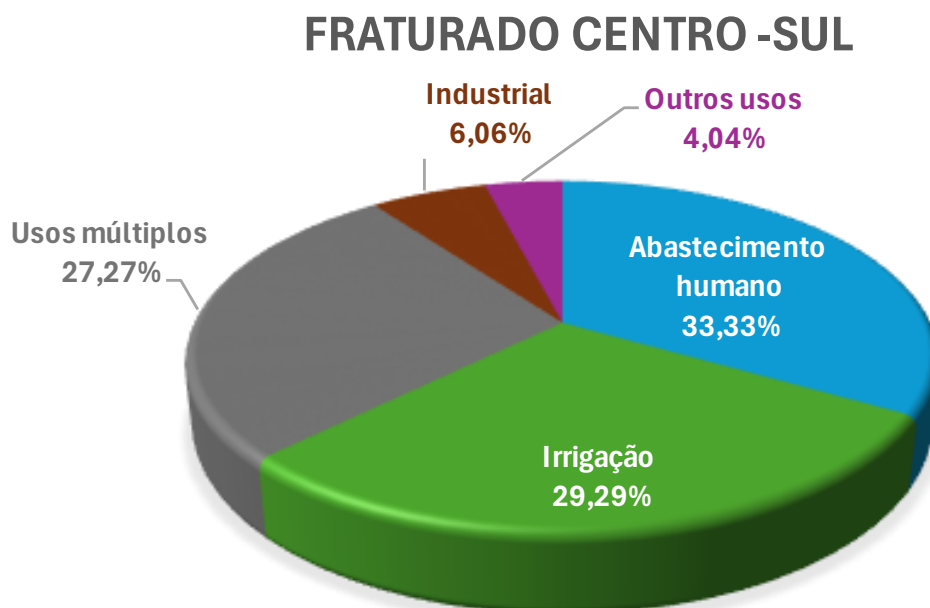
Figura 4.93 - Percentual por tipo de uso, individualizados por Sistema Aquífero - Fraturado Centro-Sul
