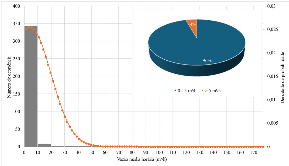
Figura 4.89 - Histograma log normal da vazão média horária para os poços do Sistema Aquífero Litorâneo Nordeste-Sudeste
