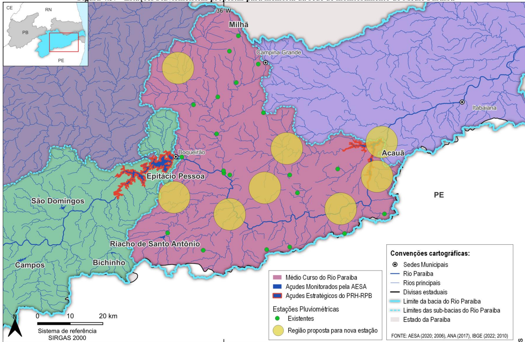
Figura 4.37 - Estações Pluviométricas propostas para melhoria da rede de monitoramento do Médio Paraíba
