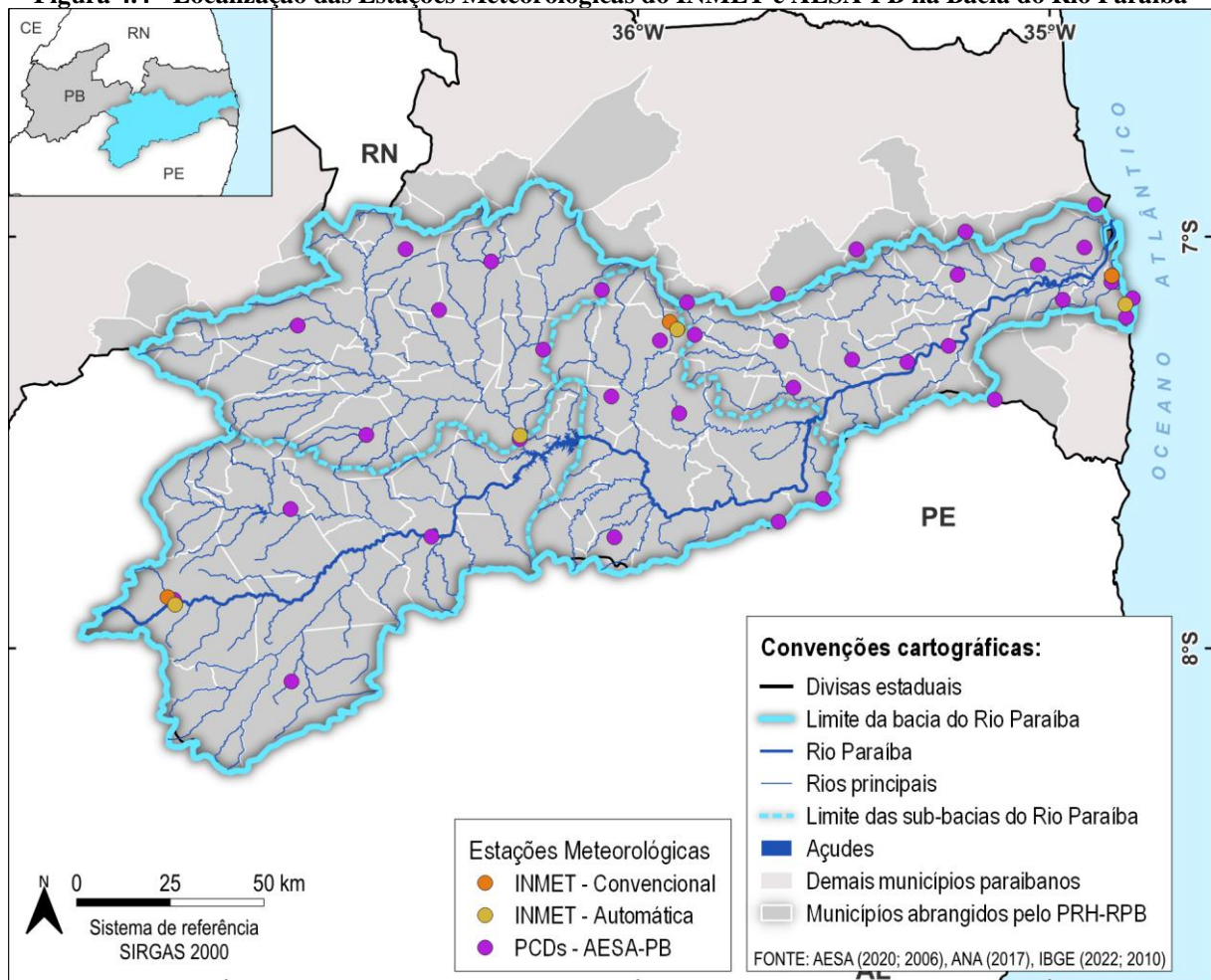
Figura 4.4 - Localização das Estações Meteorológicas do INMET e AESA-PB na Bacia do Rio Paraíba
