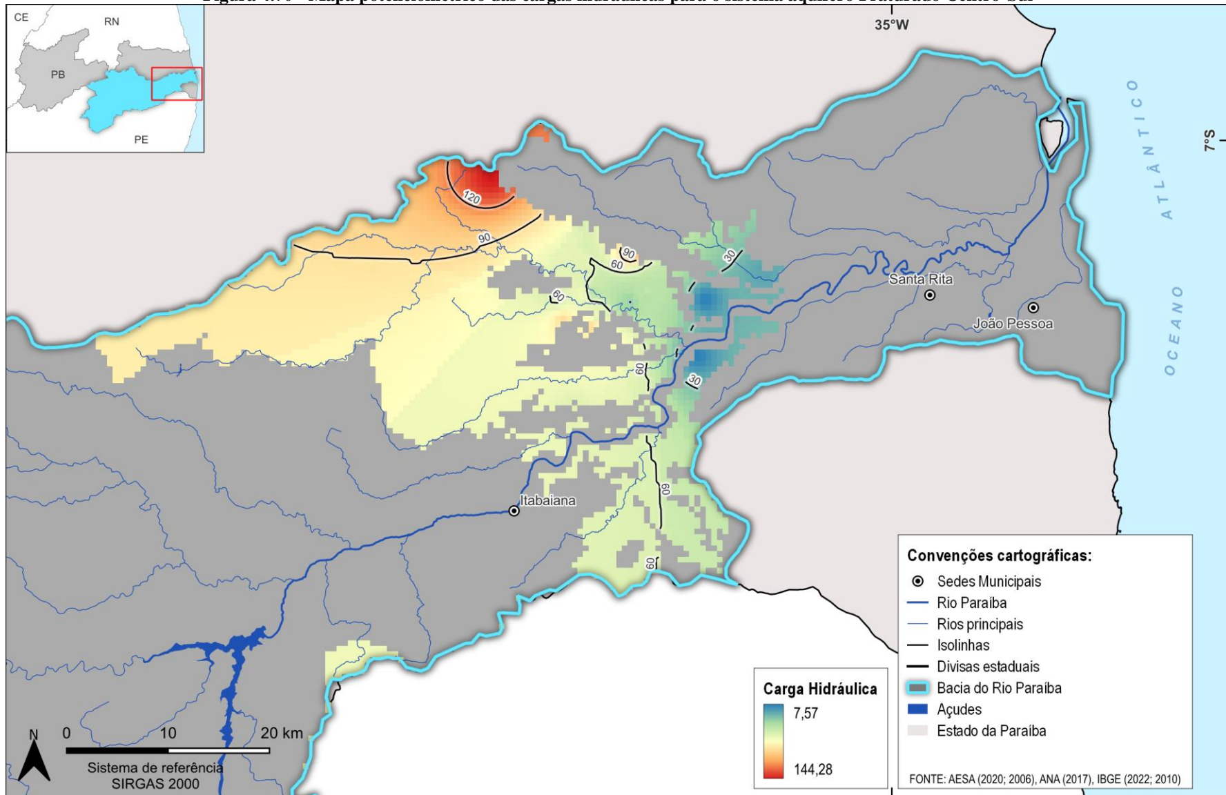
Figura 4.70 - Mapa potenciométrico das cargas hidráulicas para o sistema aquífero Fraturado Centro-Sul
