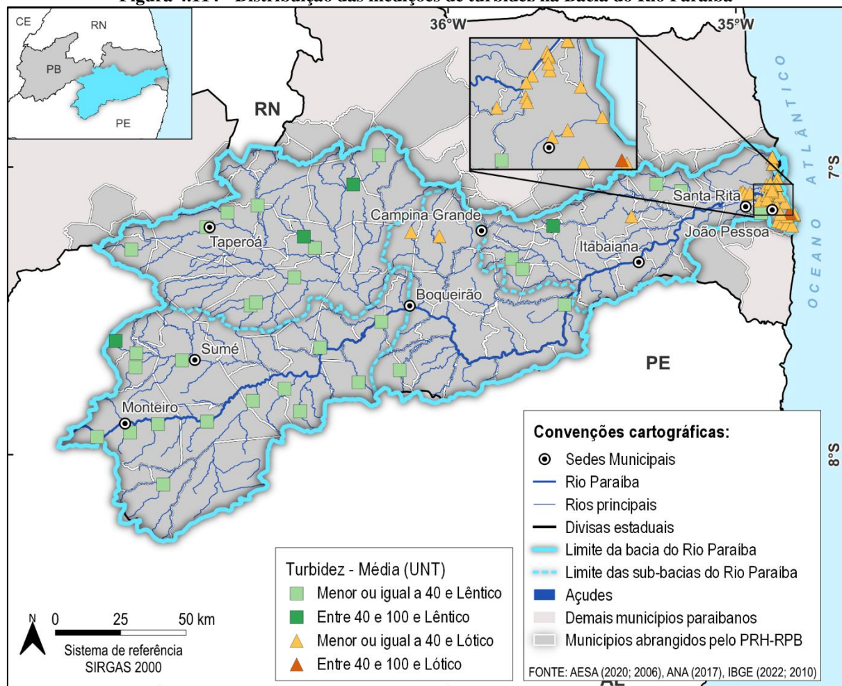
Figura 4.114 - Distribuição das medições de turbidez na Bacia do Rio Paraíba
