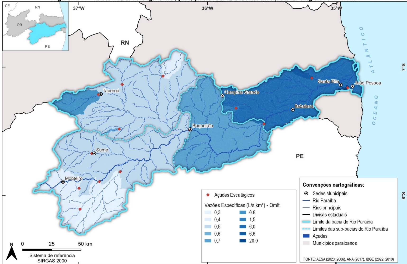
Figura 4.141 - Vazões médias de longo termo (Qmlt) para as bacias afluentes dos açudes estratégicos do PRH-RPB
