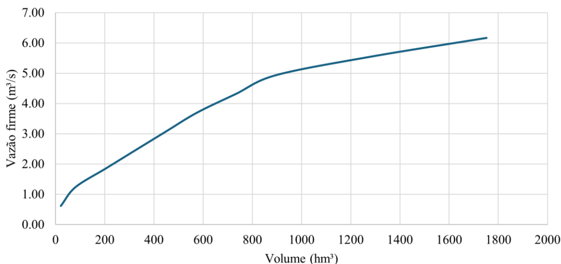
Figura 4.63 - Curva de Regularização do Açude Epitácio Pessoa
