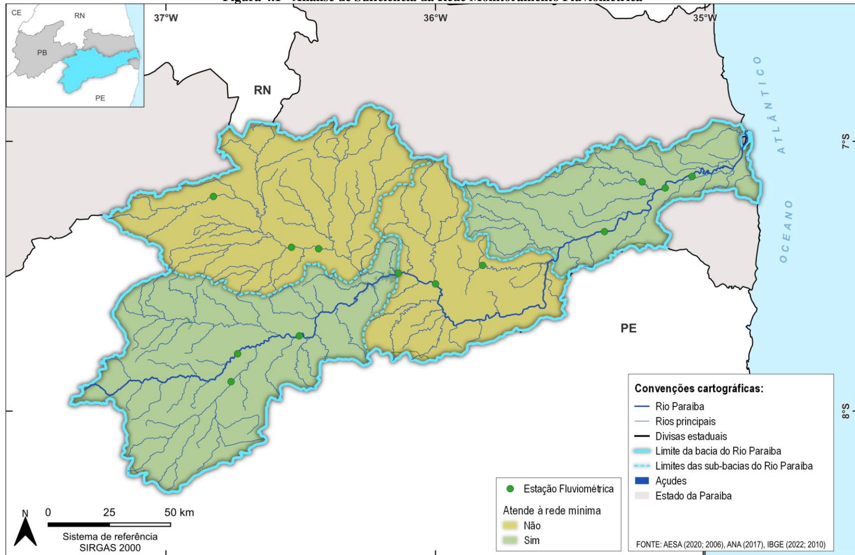
Figura 4.1 - Análise de Suficiência da Rede Monitoramento Fluviométrica
