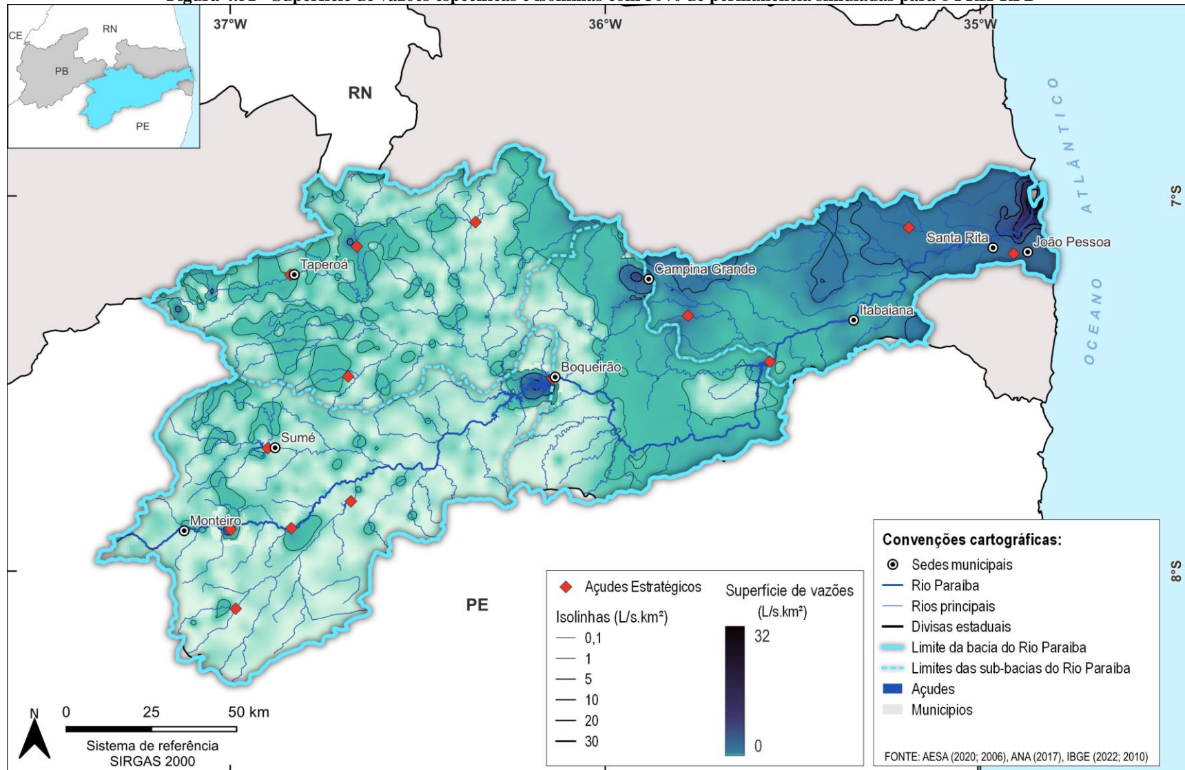
Figura 4.51 - Superfície de vazões específicas e isolinhas com 30% de permanência simuladas para o PRH-RPB
