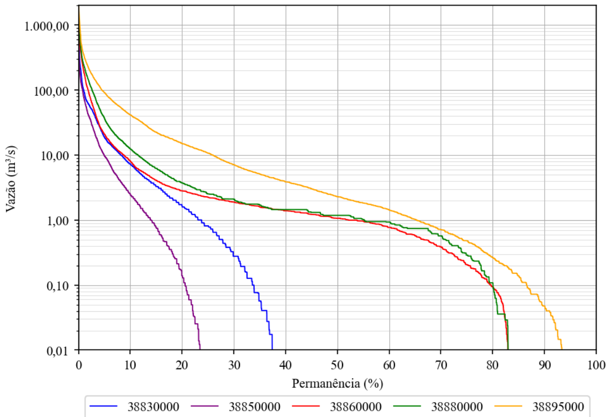
Figura 4.27 - Curvas de permanência para as Estações Fluviométricas na Bacia do Rio Paraíba
