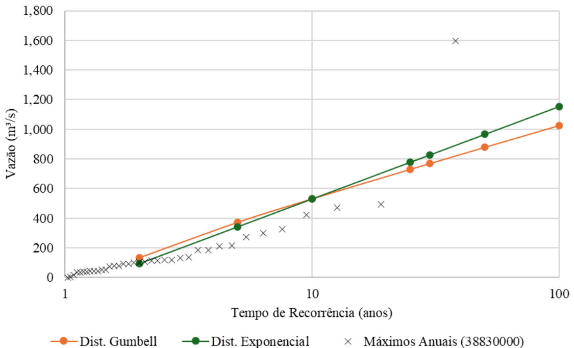
Figura 4.29 - Ajuste das distribuições de Gumbel e Exponencial para a estação 38830000
