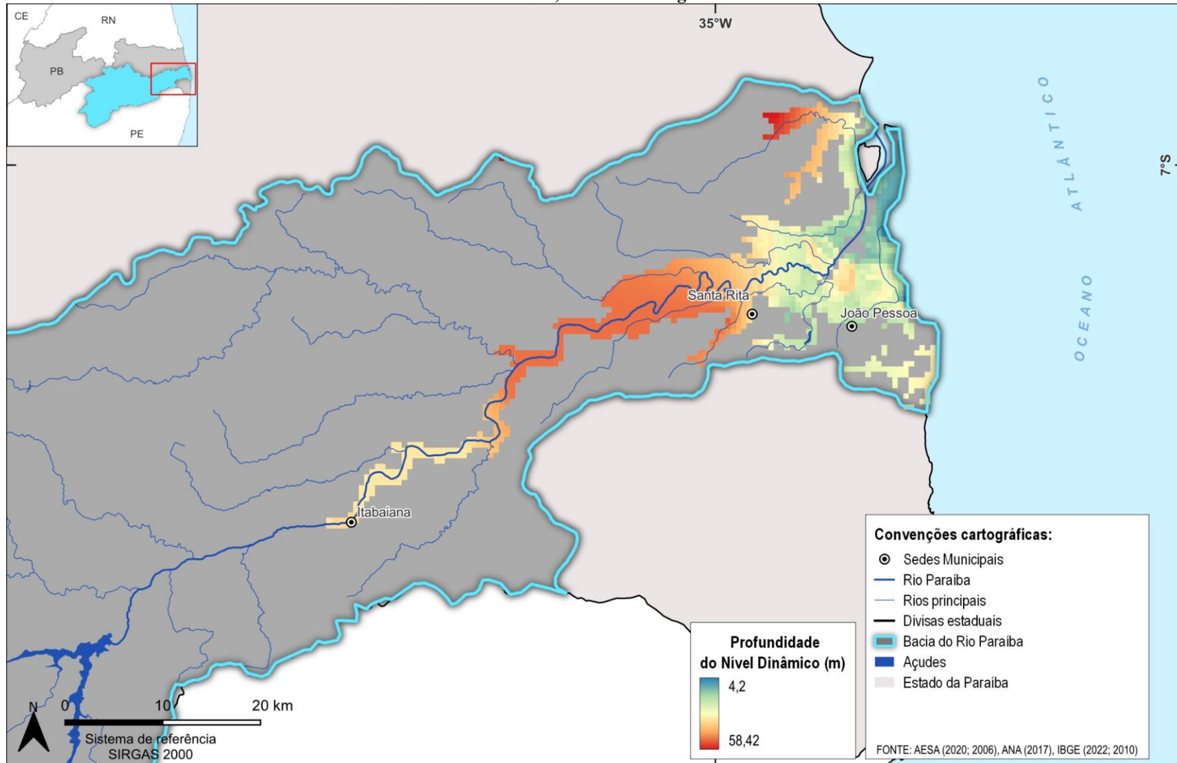
Figura 4.81 - Superfície Potenciométrica representando as Cotas (em relação ao nível médio do mar) dos Níveis Dinâmicos dos poços tubulares do sistema aquífero Litorâneo Nordeste-Sudeste, na bacia hidrográfica do Rio Paraíba
