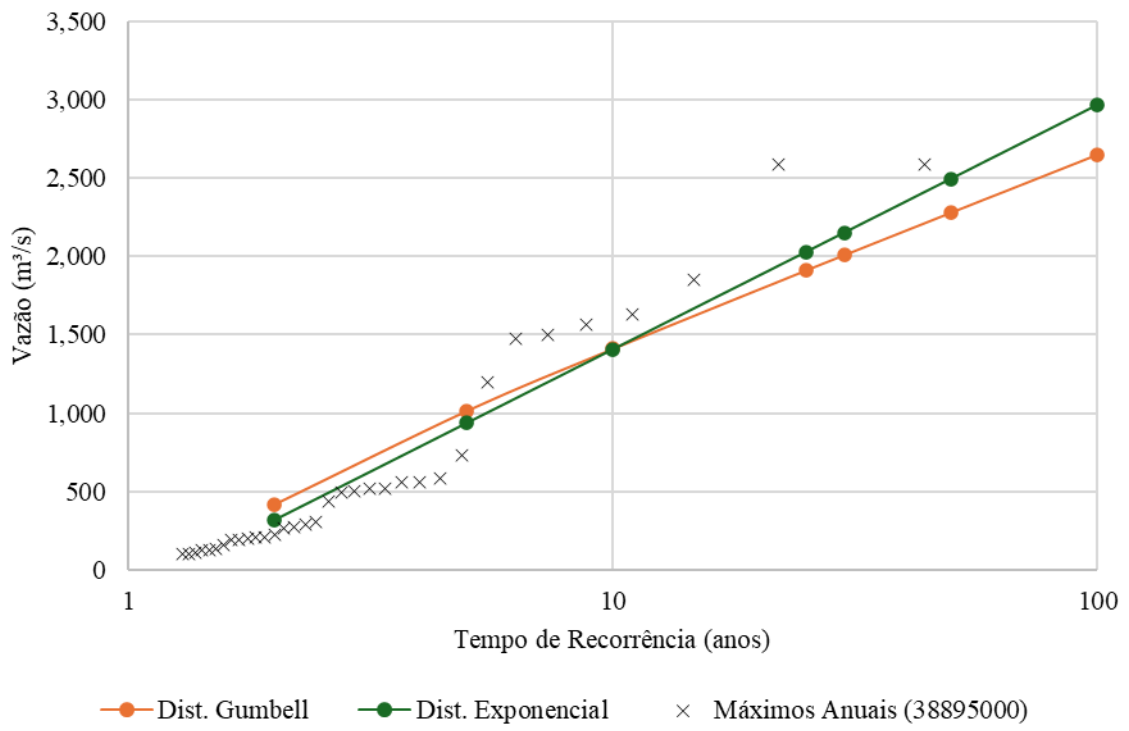
Figura 4.33 - Ajuste das distribuições de Gumbell e Exponencial para a estação 38895000
