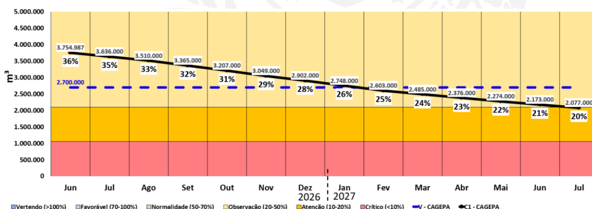
Figura 1 - Comportamento esperado do volume da barragem Catolé I.
