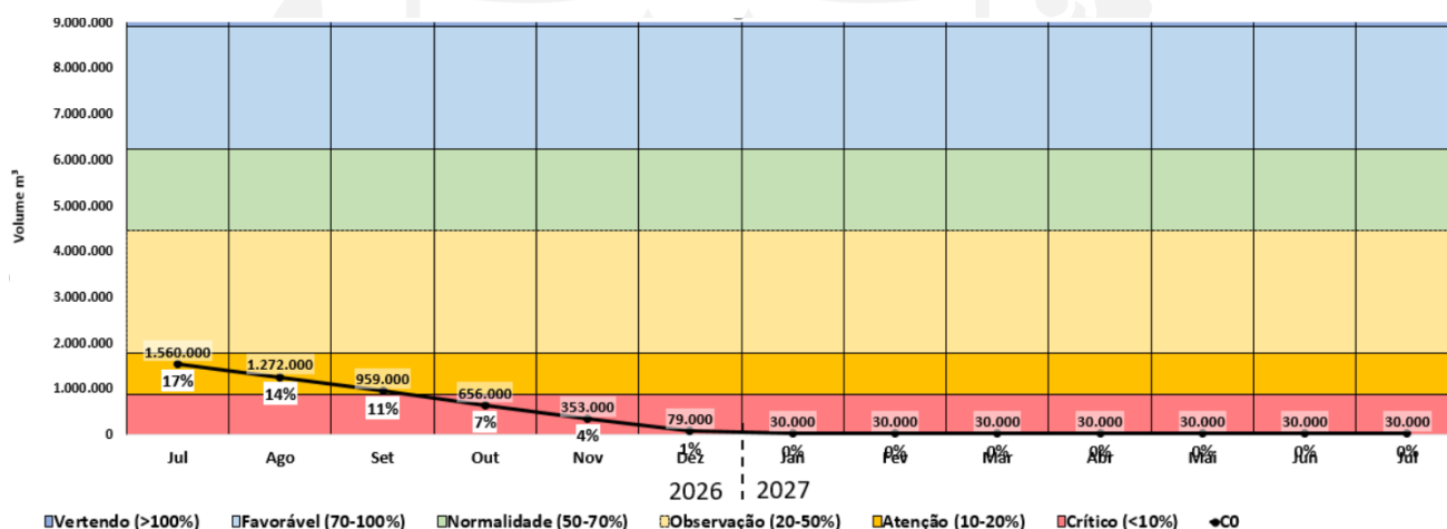
Figura 1 - Comportamento esperado do volume na barragem POÇO REDONDO.
