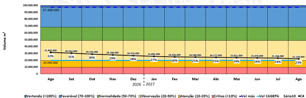
Figura 1 - Comportamento esperado do volume na barragem SACO.
