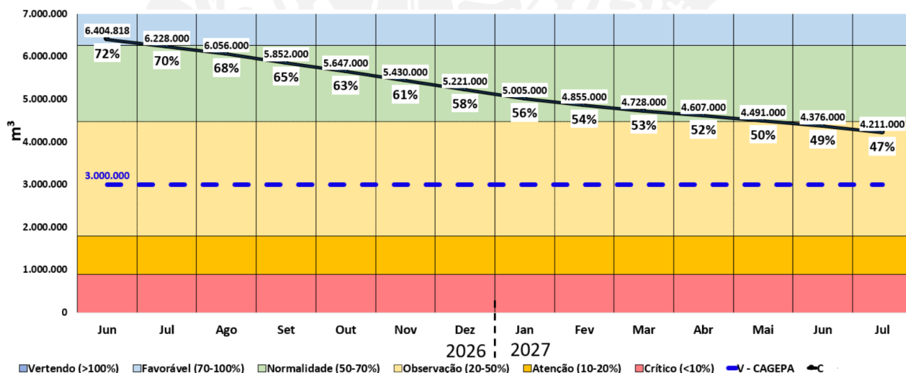
Figura 1 - Comportamento esperado do volume na barragem TAVARES II.
